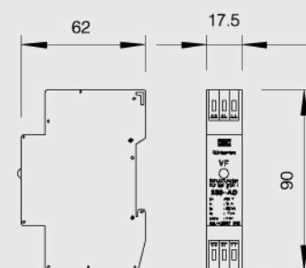
尺寸图
